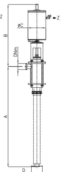
PA 140A - L con tubo de succión
