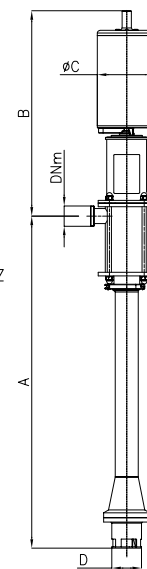
PA 140A - L con válvula de aspiración de fondo
